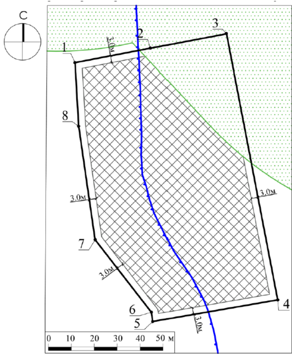
Рисунок 2 – Чертеж градостроительного плана земельного участка
